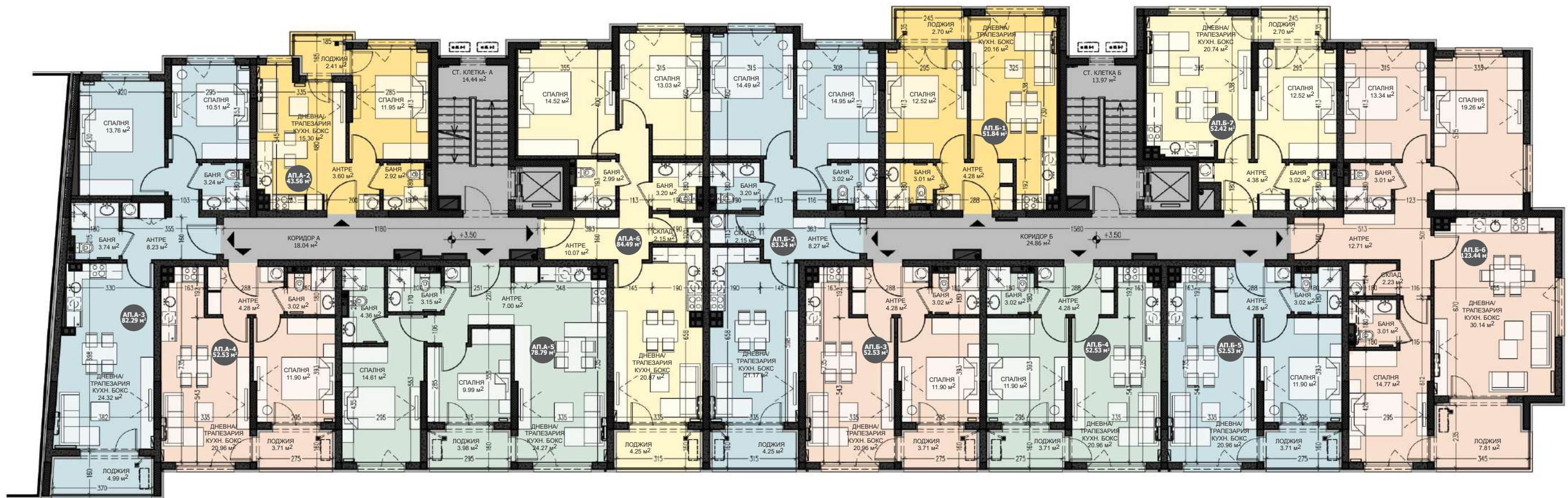
НИВО ДВЕ / КОТА +3.50
